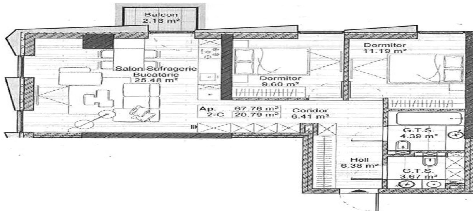
Schema amplasării apartamentului la etaj 6
